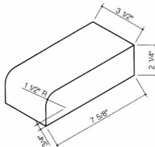
103- Bullnose Header
