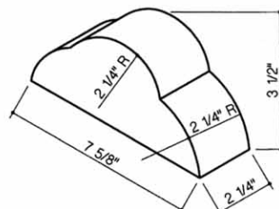
610-Wall Cap
