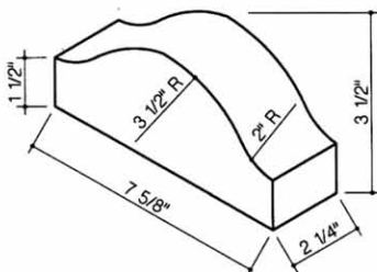
510-Wall Cap
