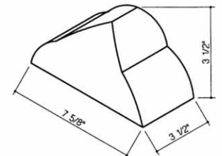
611-Wall Cap End
